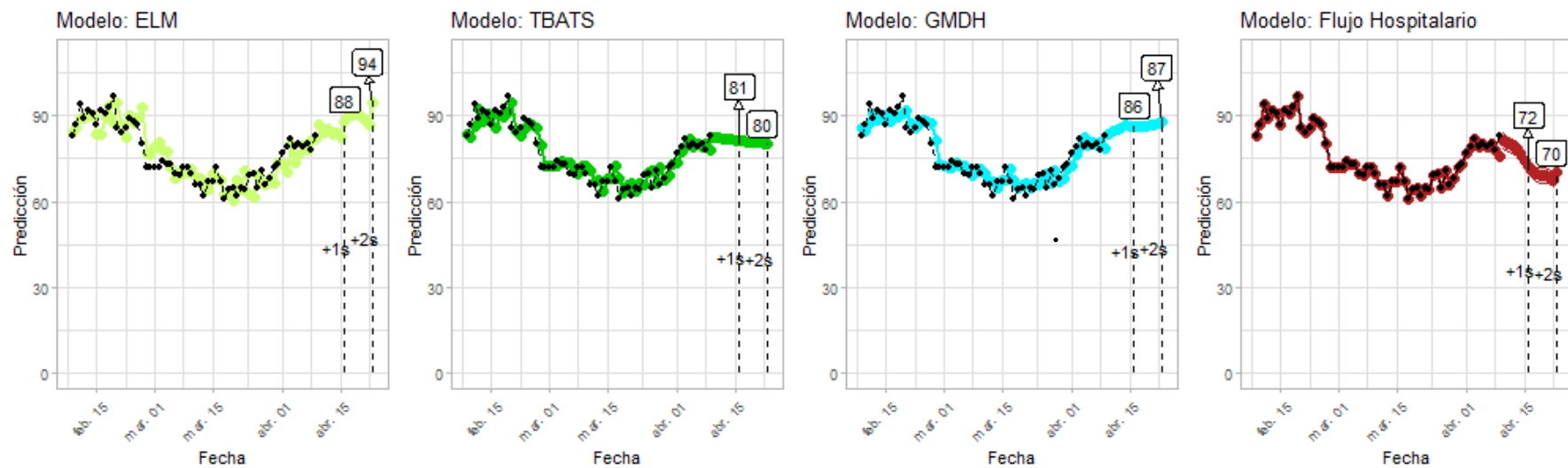
Figura 28: Predicciones de cuatro modelos – Los Lagos
