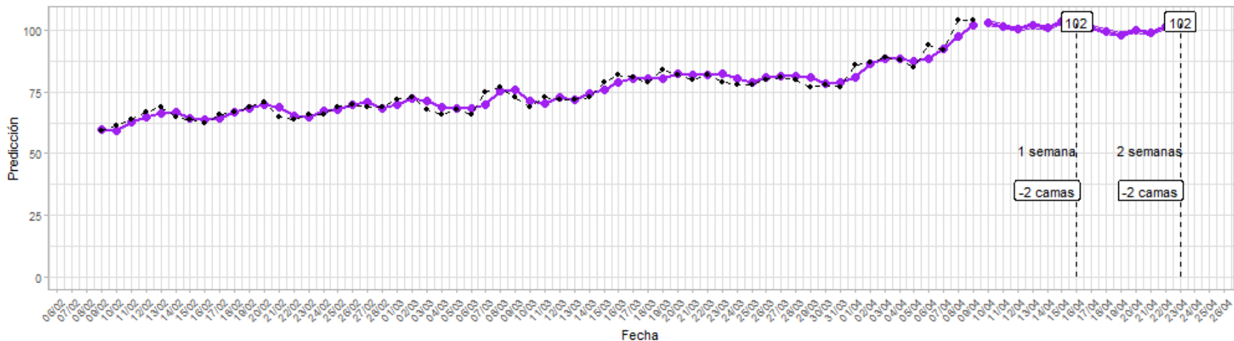
Figura 23: Mejor predicción basada en cuatro modelos - Araucanía
