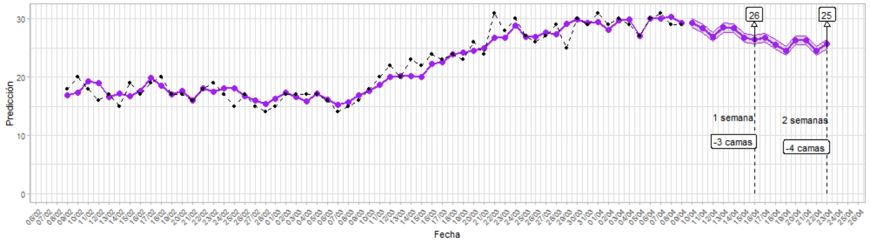
Figura 25: Mejor predicción basada en cuatro modelos – Los Ríos
