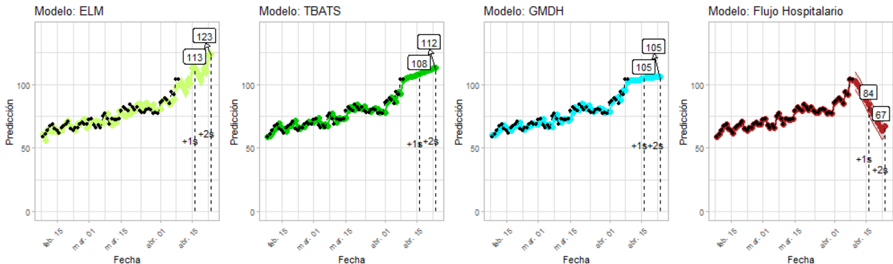
Figura 24: Predicciones de cuatro modelos - Araucanía
