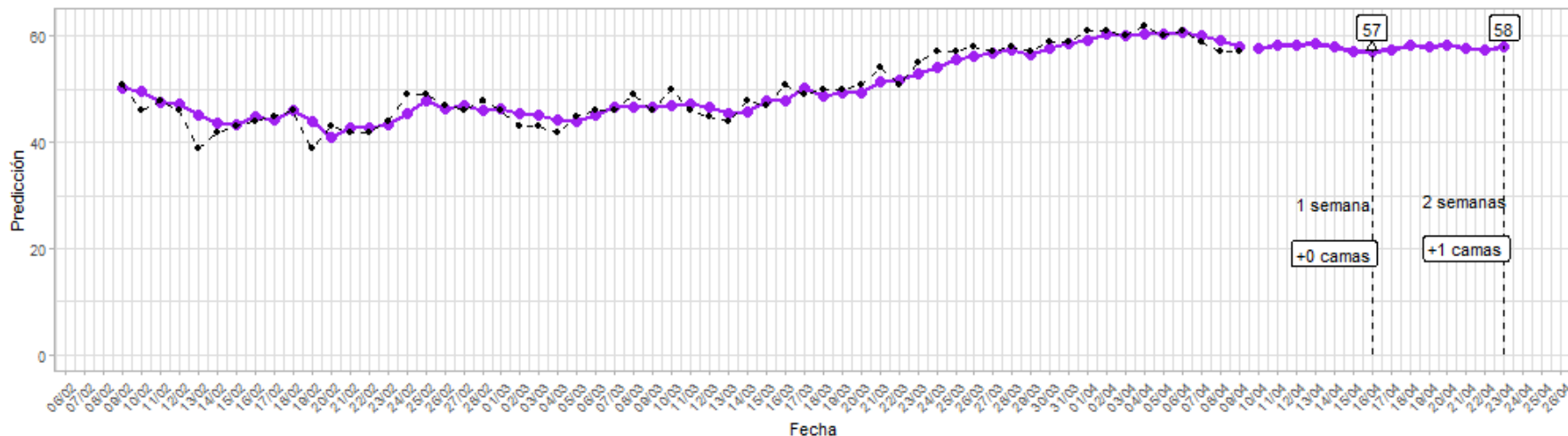
Figura 6: Predicciones de cuatro modelos - Tarapacá
