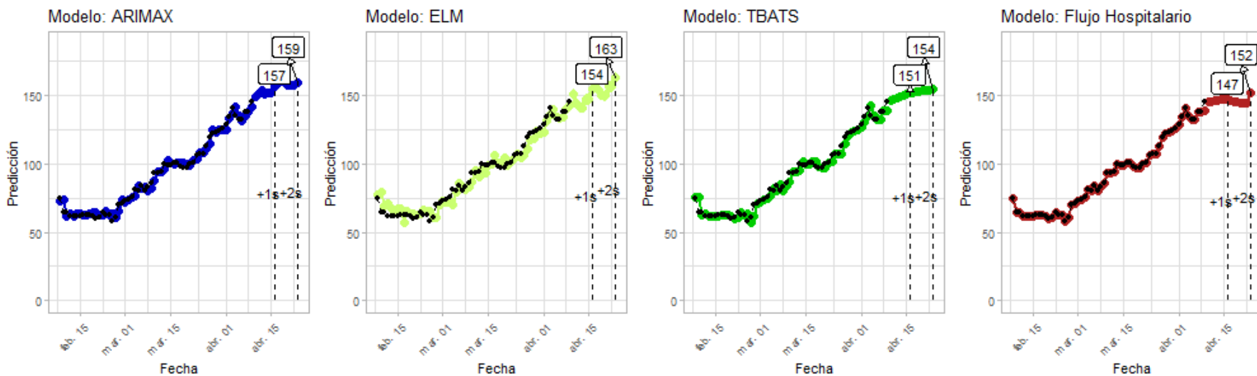
Figura 16: Predicciones de cuatro modelos – O’Higgins
