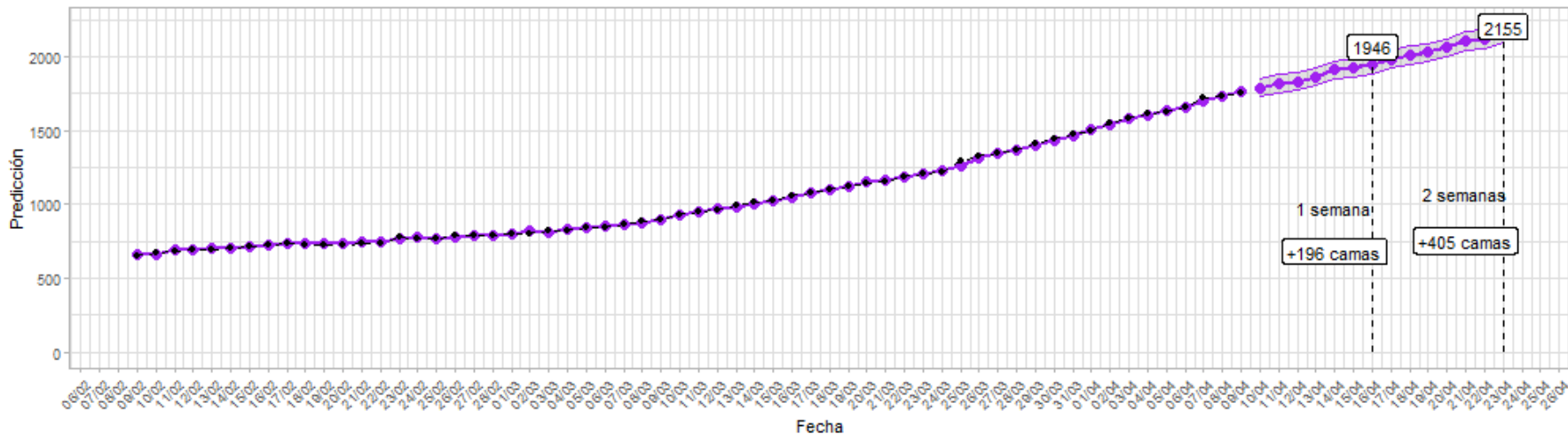
Figura 2: Predicciones de cuatro modelos - RM
