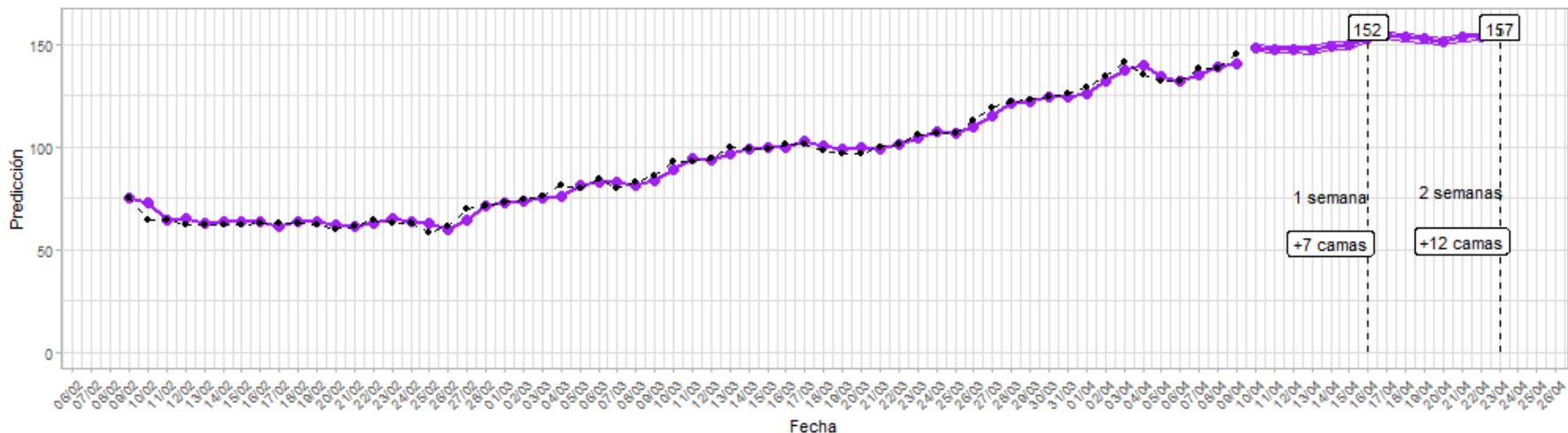
Figura 16: Predicciones de cuatro modelos – O’Higgins
