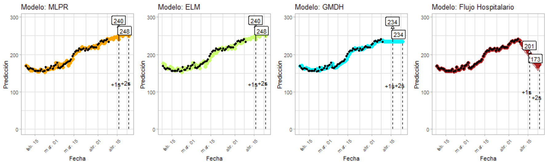
Figura 22: Predicciones de cuatro modelos - Biobío
