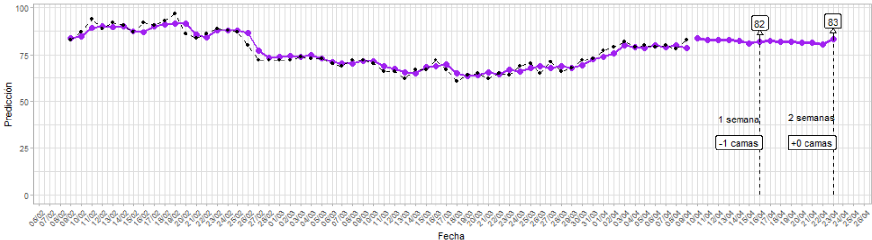
Figura 28: Predicciones de cuatro modelos – Los Lagos
