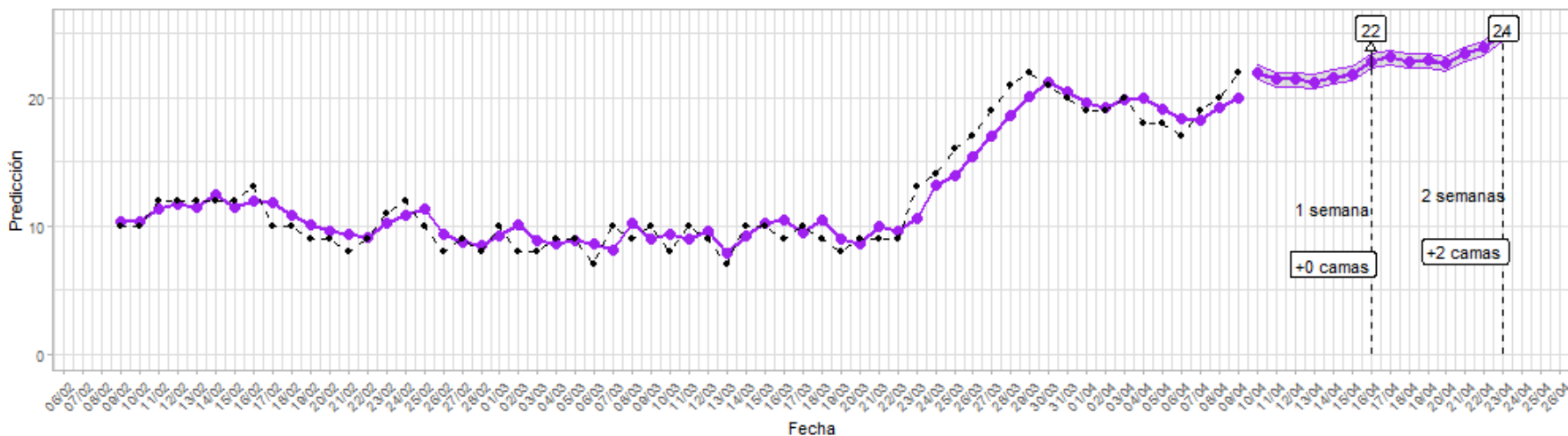
Figura 9: Mejor predicción basada en cuatro modelos - Atacama
