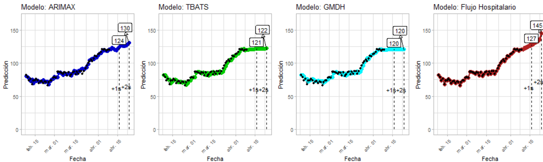
Figura 18: Predicciones de cuatro modelos - Maule
