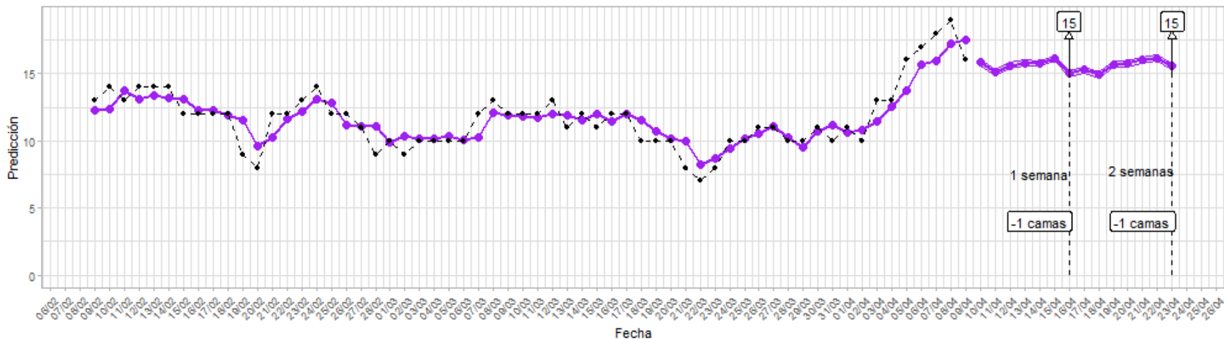
Figura 32: Predicciones de cuatro modelos - Magallanes
