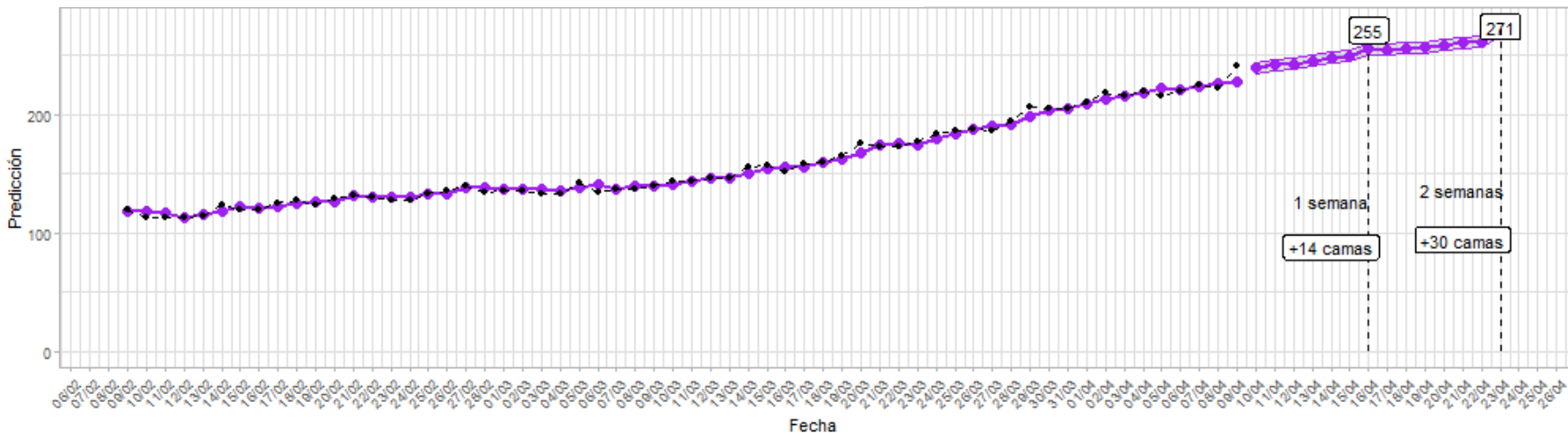
Figura 13: Mejor predicción basada en cuatro modelos - Valparaíso
