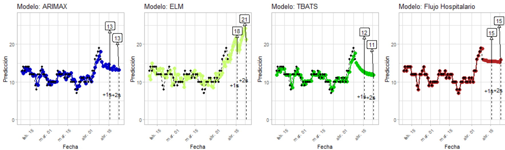
Figura 32: Predicciones de cuatro modelos - Magallanes
