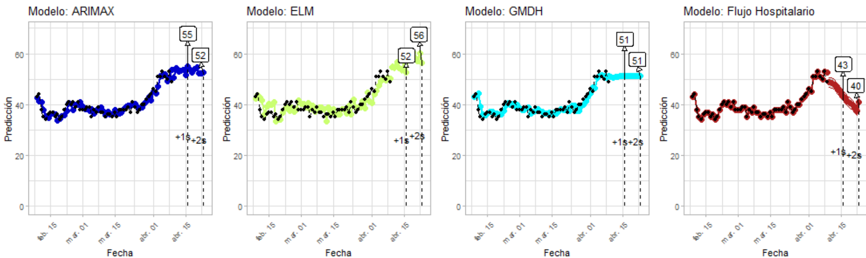
Figura 20: Predicciones de cuatro modelos - Ñuble
