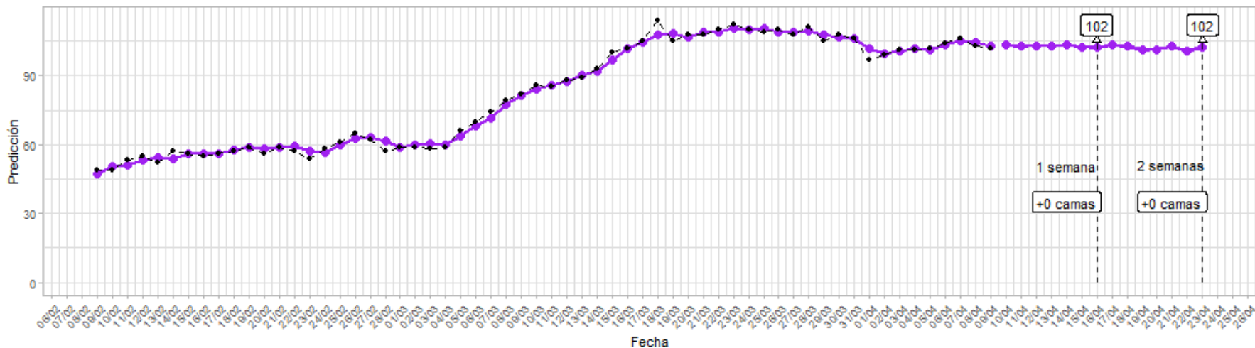
Figura 12: Predicciones de cuatro modelos - Coquimbo
