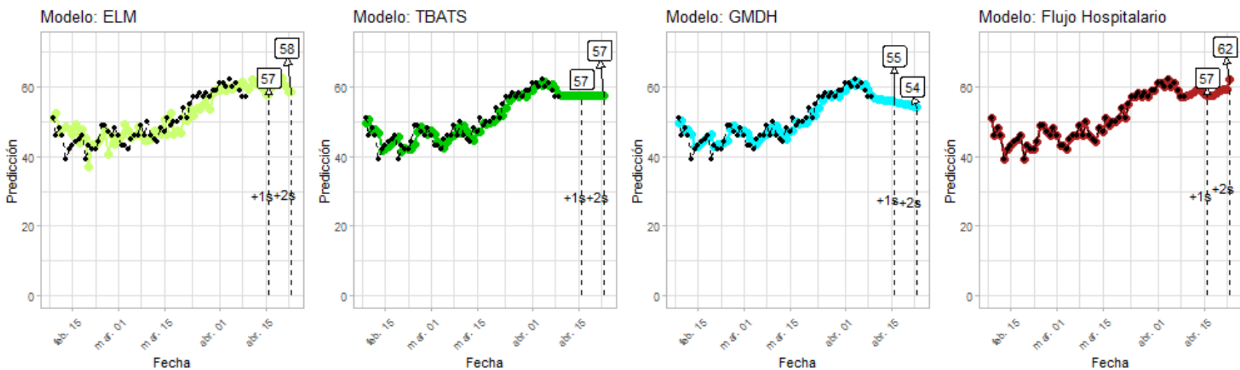
Figura 6: Predicciones de cuatro modelos - Tarapacá
