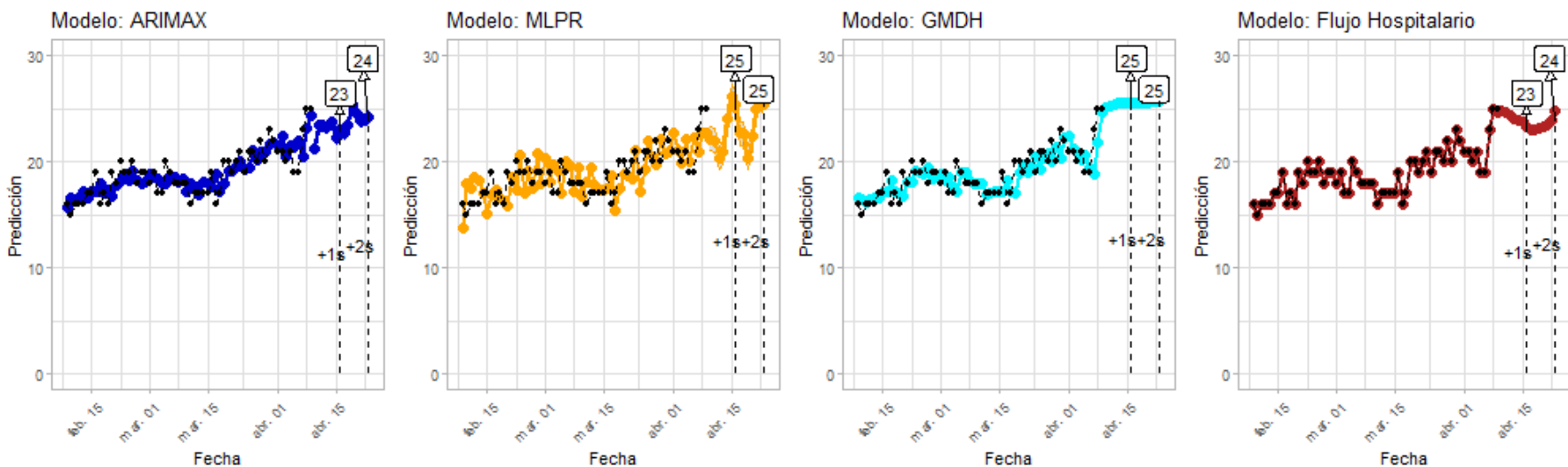
Figura 4: Predicciones de cuatro modelos – Arica y Parinacota
