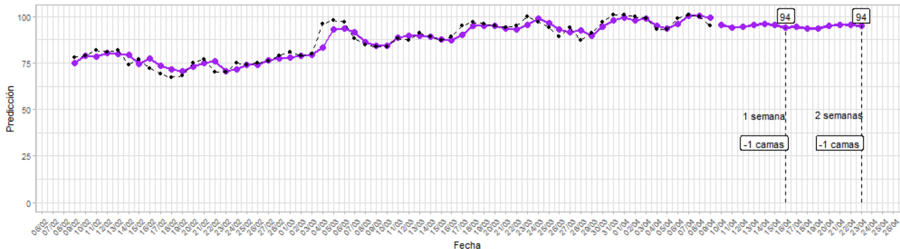
Figura 8: Predicciones de cuatro modelos - Antofagasta
