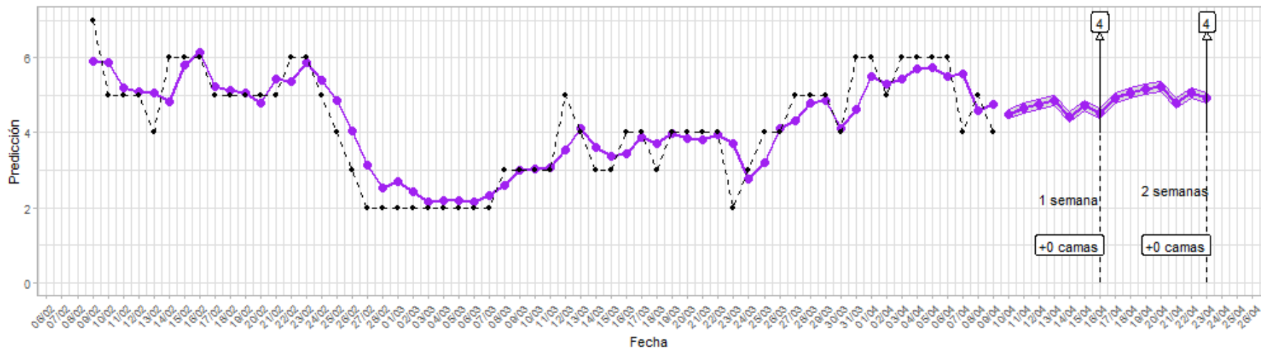
Figura 30: Predicciones de cuatro modelos - Aysén
