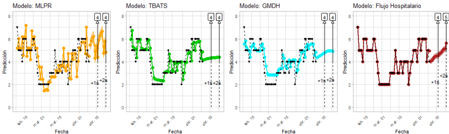
Figura 30: Predicciones de cuatro modelos - Aysén
