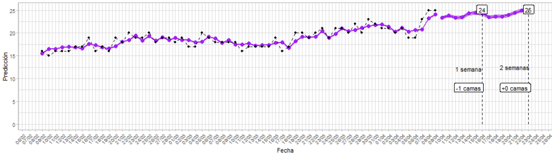
Figura 4: Predicciones de cuatro modelos – Arica y Parinacota
