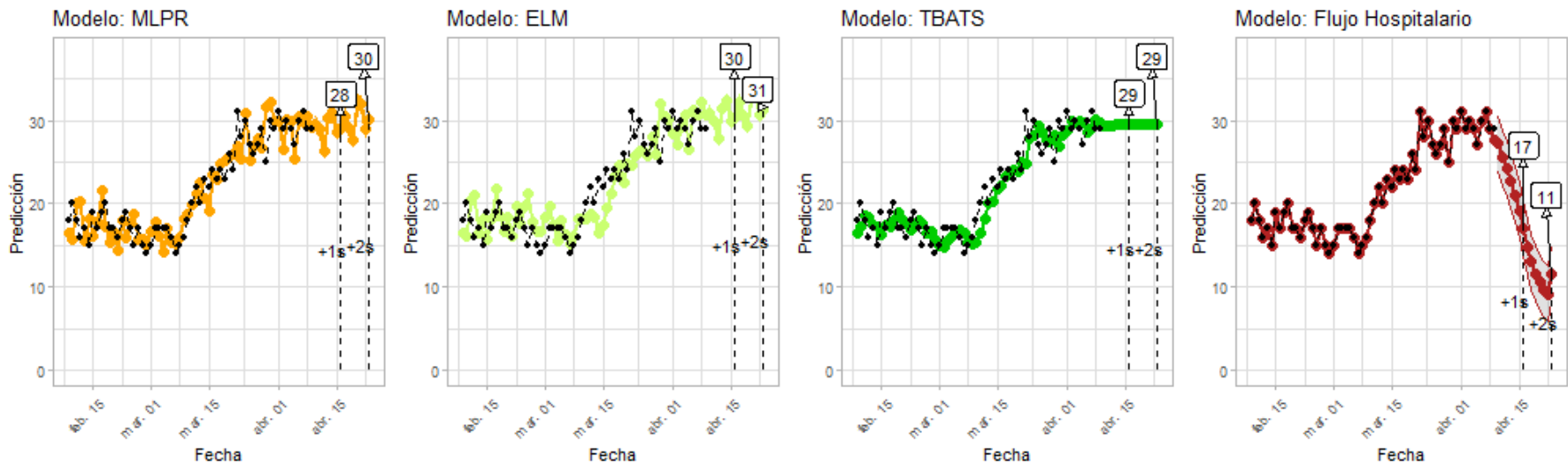
Figura 26: Predicciones de cuatro modelos – Los Ríos
