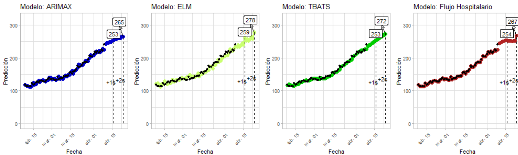
Figura 14: Predicciones de cuatro modelos - Valparaíso
