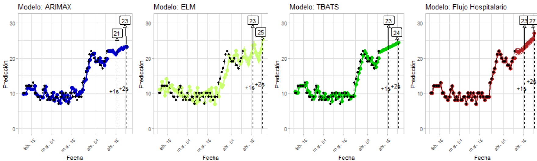
Figura 10: Predicciones de cuatro modelos - Atacama
