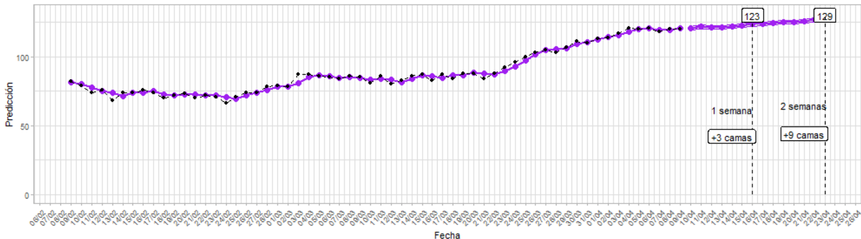
Figura 18: Predicciones de cuatro modelos - Maule
