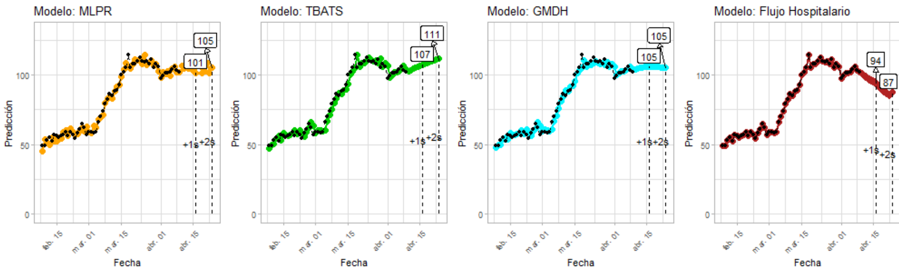
Figura 12: Predicciones de cuatro modelos - Coquimbo
