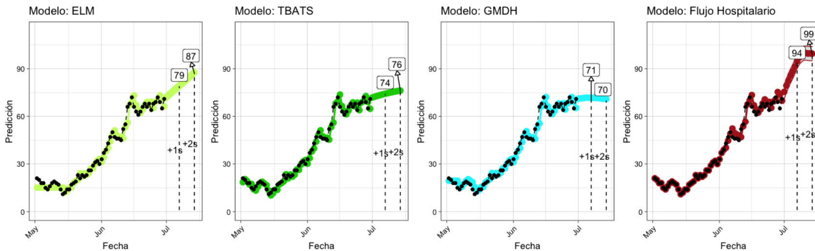
Figura 12: Predicciones de cuatro modelos – Biobío
