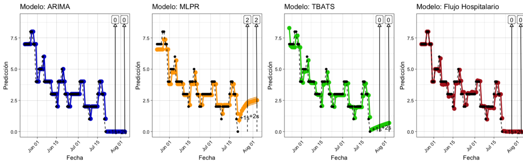
Figura 26: Predicciones de cuatro modelos – Magallanes
